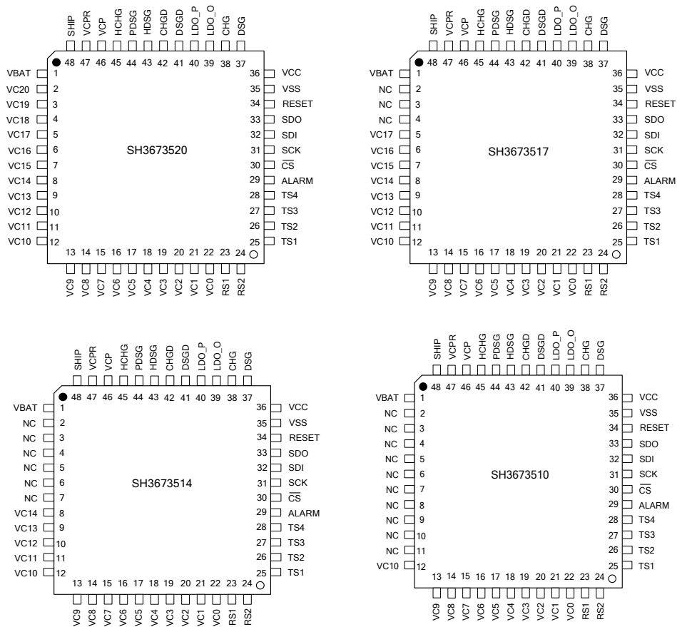
图2 管脚配置图
