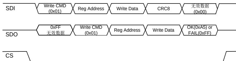
图9 寄存器写时序
