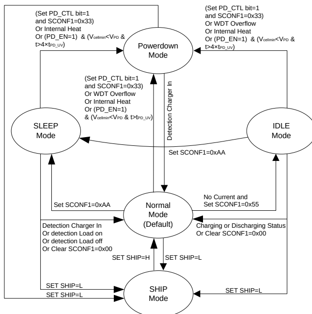
图5 模式转换图
